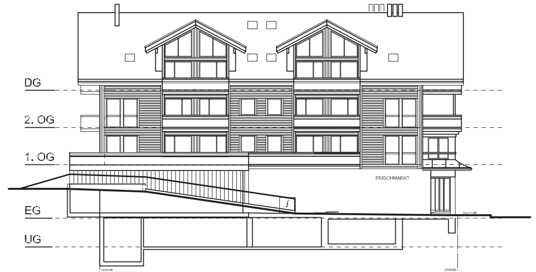
Nordansicht (Zugang Männlichenbahn)
