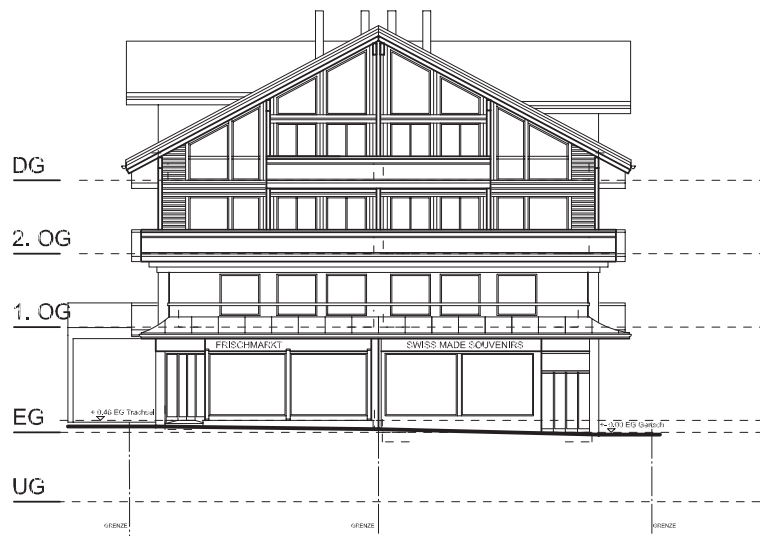
Westansicht
