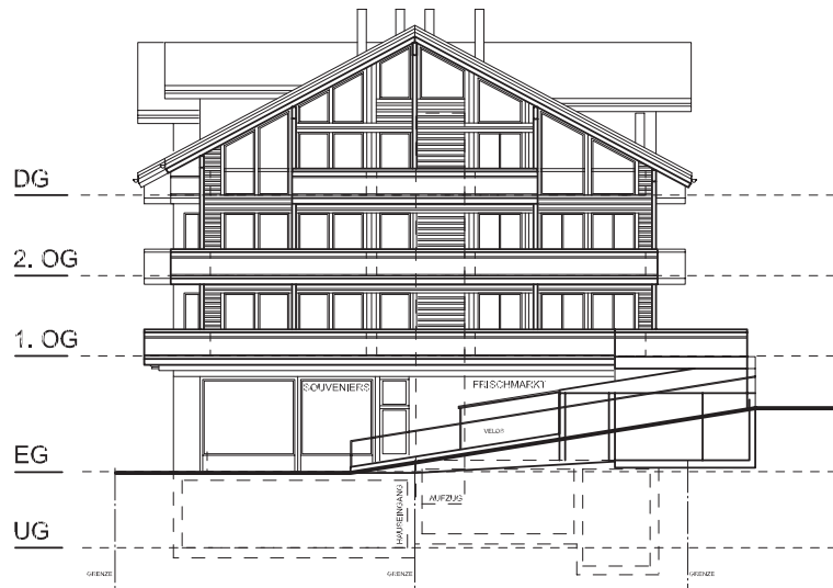
Ostansicht (Männlichenbahn)
